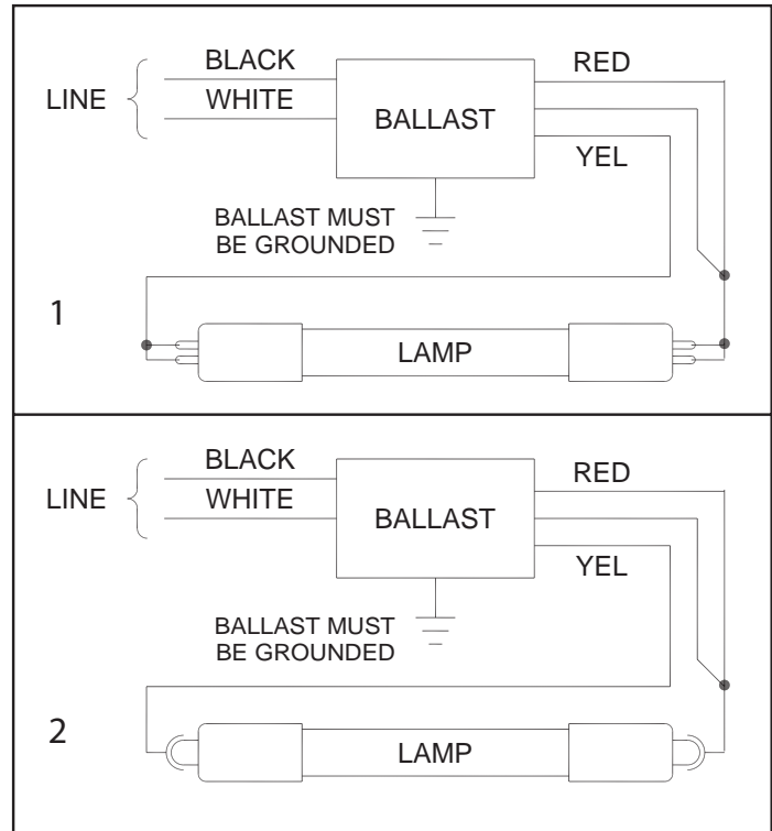
Wiring Diagrams
