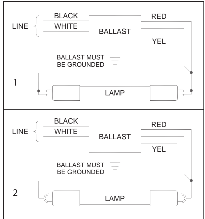
Wiring Diagrams
